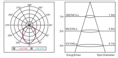
20W 85°
